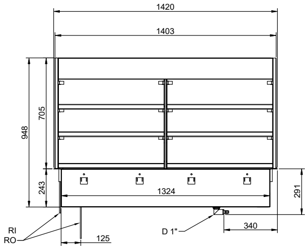
Achterzijde
